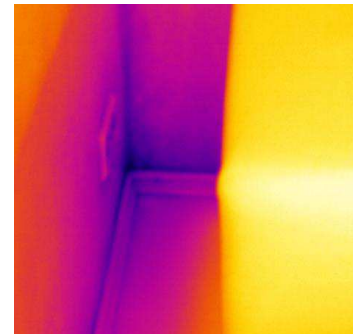
Schimmelgefahr durch Möbel an der Außenwand
