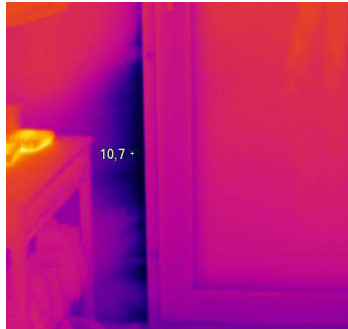
Luftundichtigkeiten bei einer Außentür
